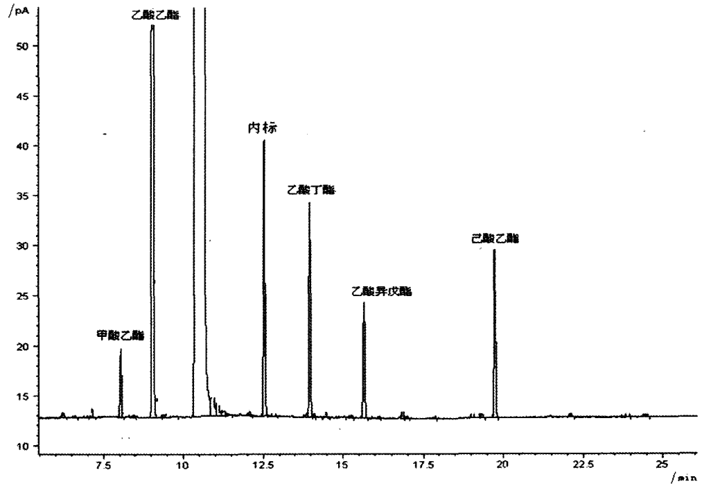
图A.1 5种酯标准品的色谱图
