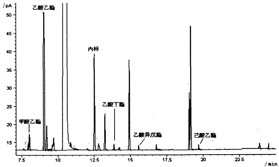
图A.2 黄酒样品中5种酯的色谱图
